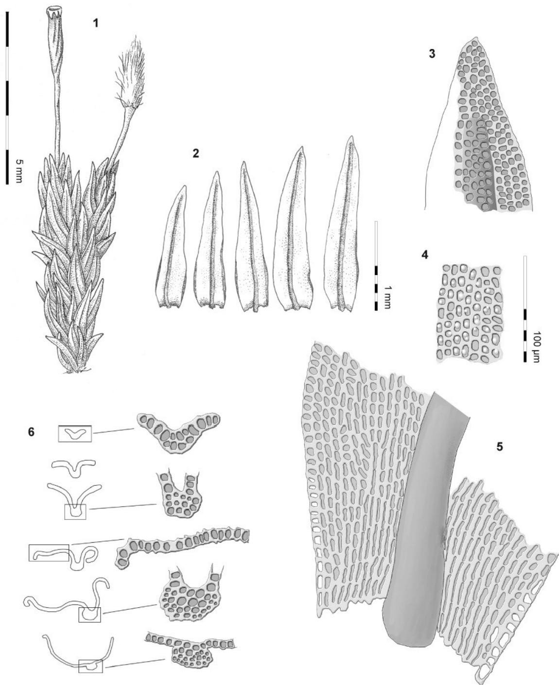
Abb. 1 Ulota hutchinsiae (Sm.) Hammar. 1: Habitus. 2: Blätter. 3: Apikale Blattzellen. 4: Mittlere Blattzellen. 5: Basale Blattzellen. 6: Blattquerschnitte.
