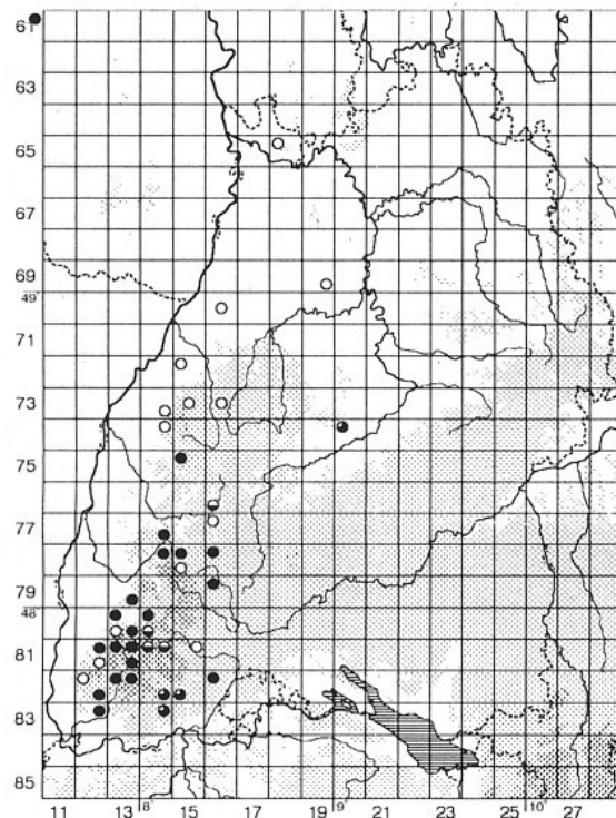
Abb. 2: Verbreitung von Ulota hutchinsiae in Baden-Württemberg.
